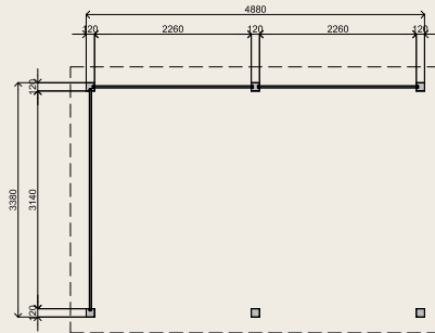
Middelburg
