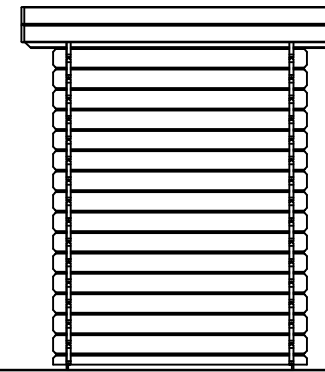
(L) Zijaanzicht / Side view / Seiten ansicht
