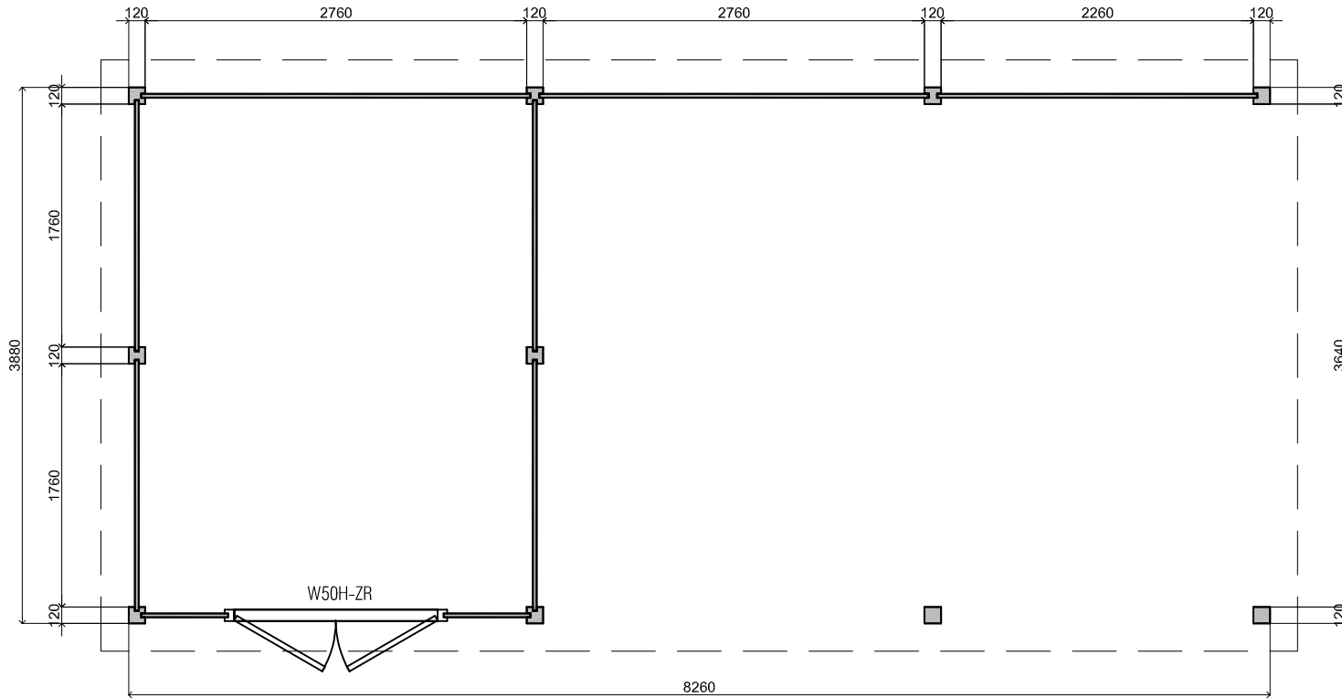
Plattegrond / Plan
