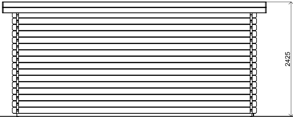
Achteraanzicht / Rear view / Hinterseite
