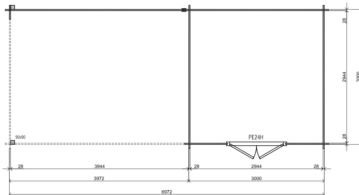
Plattegrond / Plan
